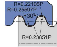
DIN 405 Tolerance: 7
