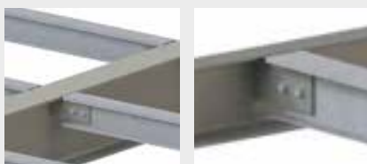
IPE-Profil
